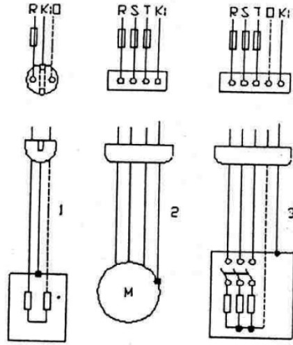
Şekil 12 - Elektrik Tüketicilerinin Sıfırlamada Fiş ve Priz Üzerinden Taşınabilir Bağlantıların Yapılması
