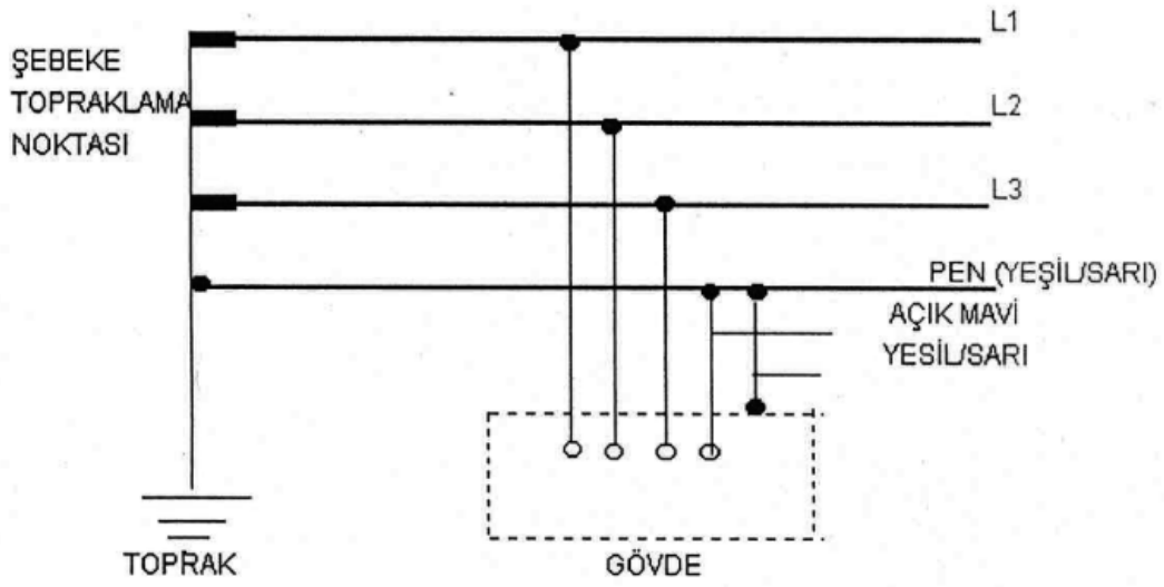
Şekil 1-1 Tümdü Korum ve Nötr İşlevlerinin Yüklendiği Tek İletken Çekilmiş TN Sistemi (TN-C)
